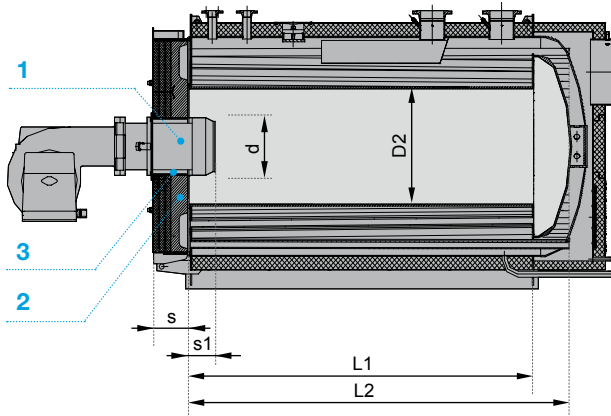
Instalación del quemador
