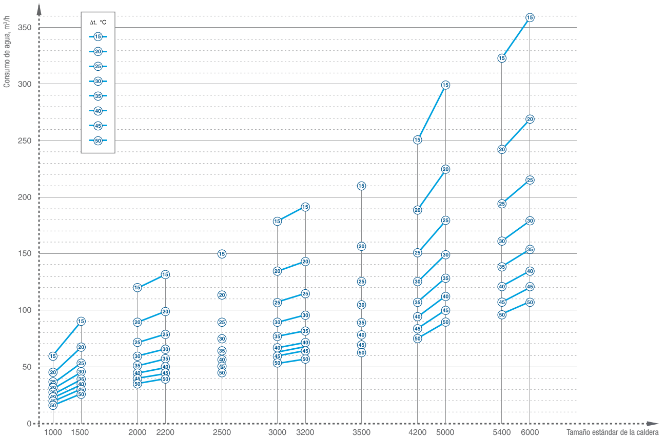
Dependencia del consumo de agua de las calderas TT100 respecto a la Δt
