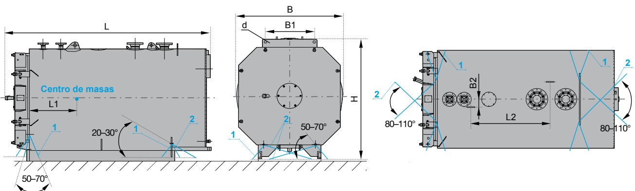
Esquema de transporte de calderas con salida de calor de 4200-20 000 KW
