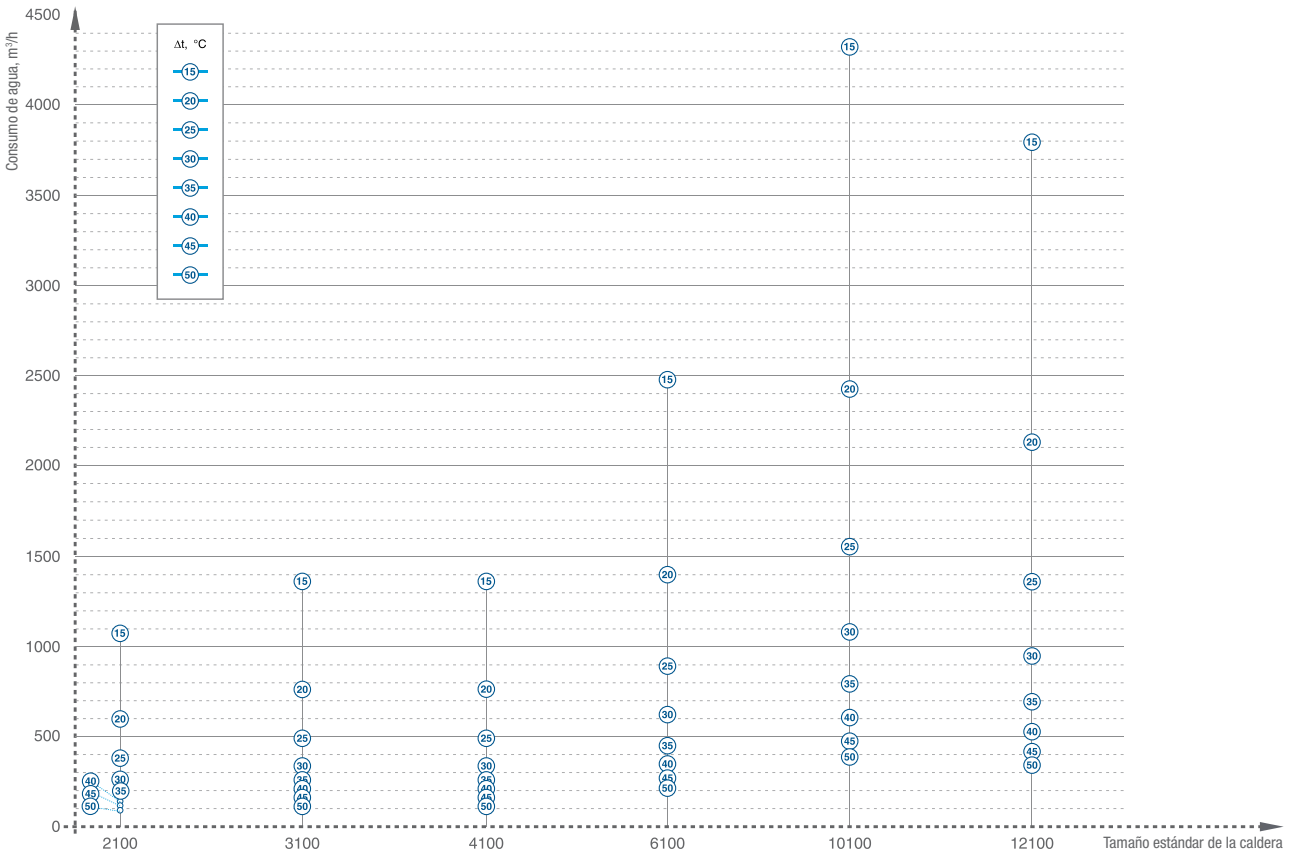
Dependencia de la resistencia hidráulica de las calderas TT100 respecto a la Δt (en modo invernal)
