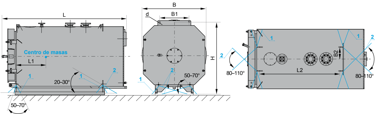
Esquema de transporte de calderas con salida de calor de 1000-3500 KW
