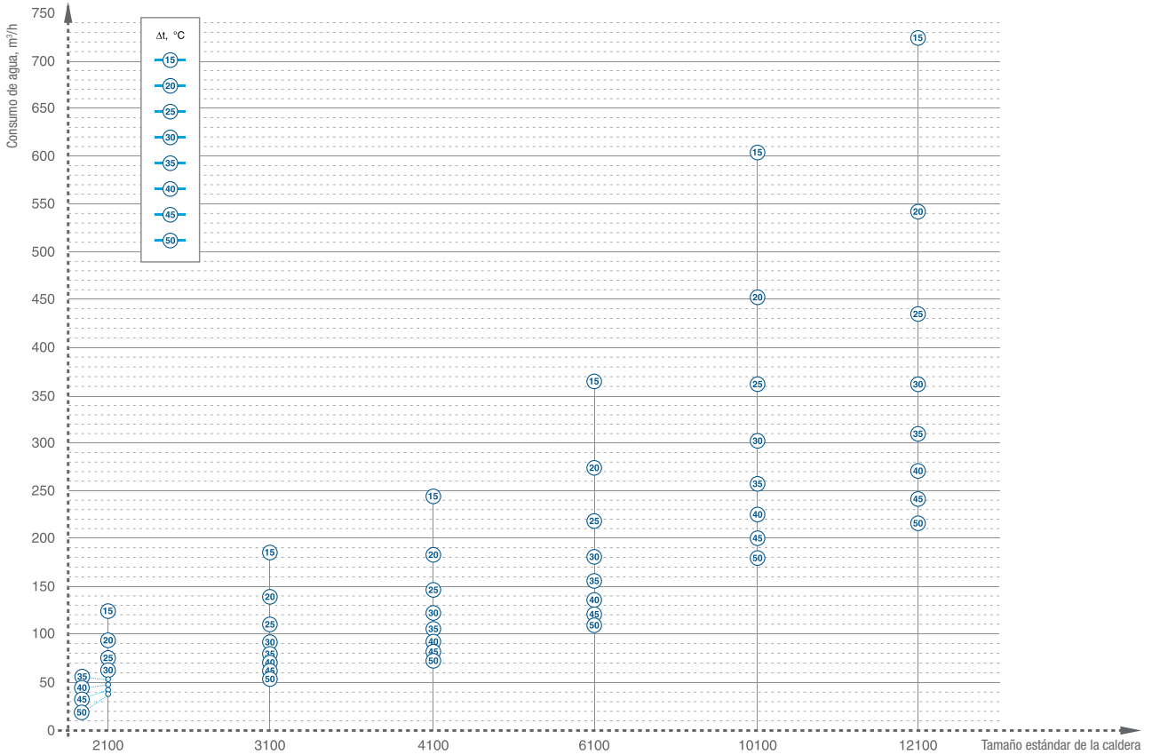
Dependencia del consumo de agua de las calderas TT100 respecto a la Δt (en modo invernal)
