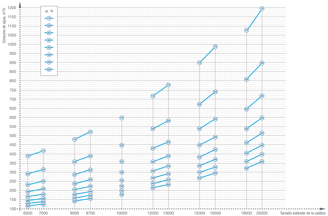
Dependencia del consumo de agua de las calderas TT100 respecto a la Δt. Continuación
