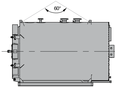
Esquema principal del eslingamiento de la caldera
