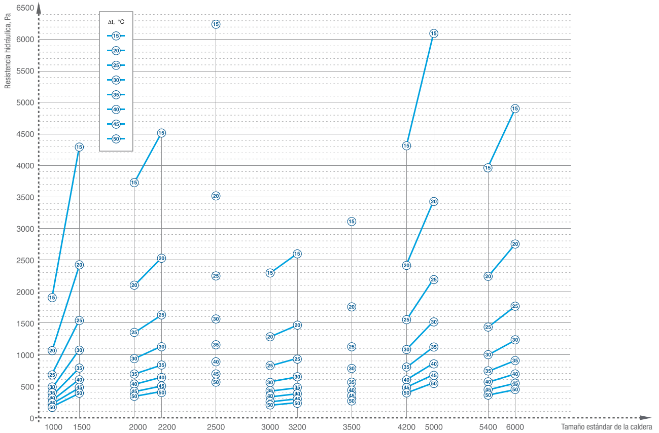
Dependencia de la resistencia hidráulica de las calderas TT100 respecto a la \Delta t .
