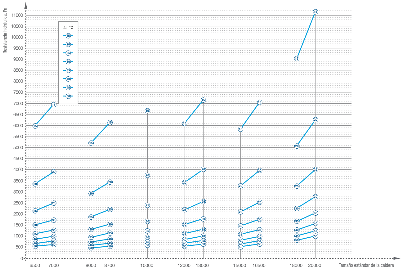
Dependencia de la resistencia hidráulica de las calderas TT100 respecto a la \Delta t . Continuación
